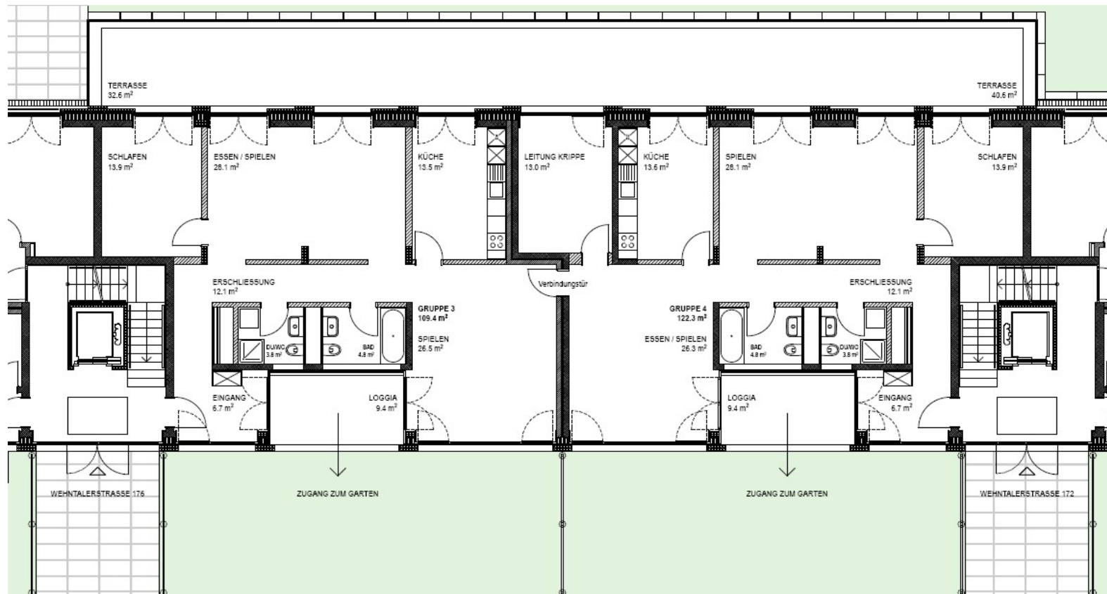
Abb. 3 Einzelne Gruppenräumlichkeiten Betreuungsgruppe Wombels und Mumins : Grundrisse
